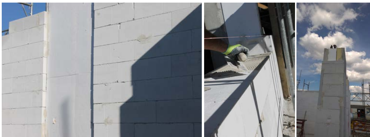
Fasi della posa dei blocchi YTONG per il tamponamento e la correzione dei ponti termici
